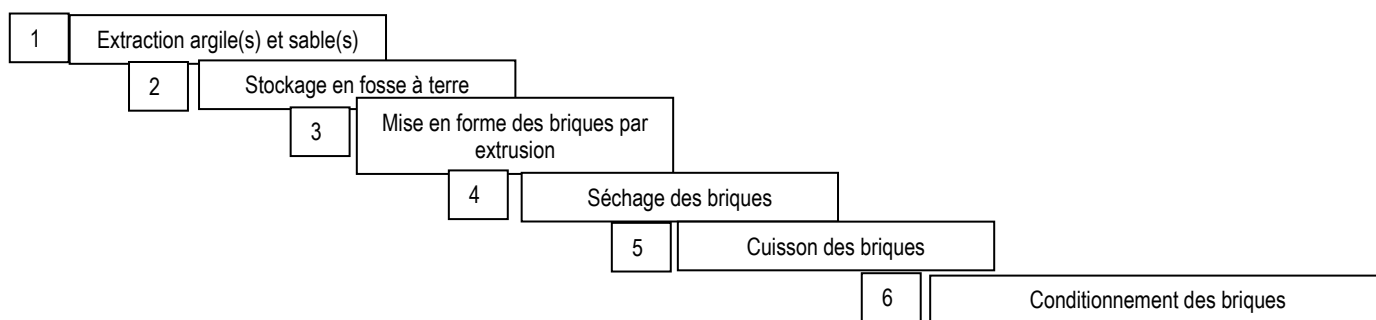
Schéma décrivant le procédé classique de fabrication des briques de 22cm x 22cm
